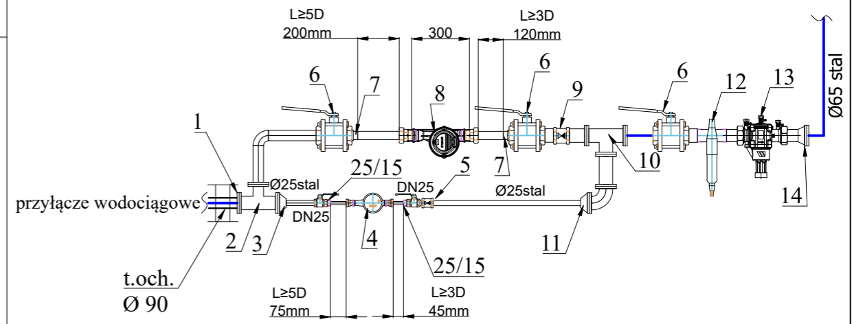
SCHEMAT ZESTAWU WODOMIERZOWEGO skala 1:50
